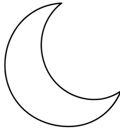
Moon
